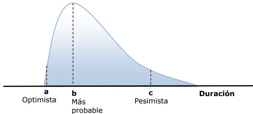
Distribución Beta
